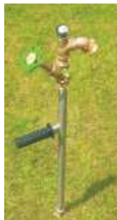
mini-ÜH Bewässerungshydrant bis 40 cbm/h -Edelstahl-
