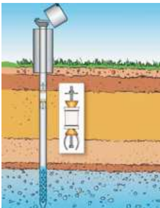
Spezial Pegelsicherung Innerer Pegelschutz, nur mit Spezialschlüssel demontierbar
