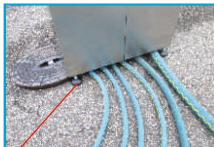
4 Höhenverstellbare Pendelfüße ermöglichen bis zu 10 cm Spalt für die Schlauchdurchführung
